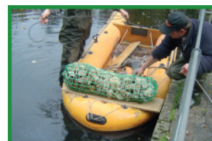
Les clôtures pour les canards se font « à sec » alors que les barrières pour les cormorans se posent une fois l'île à l'eau. Pour la fixation des îles, des sacs de pierres (0.7 à 1 m x 0.25 m) seront jetés et reliés aux angles des radeaux.
